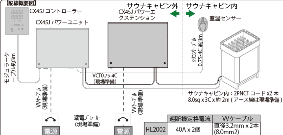
【配線概要図】
