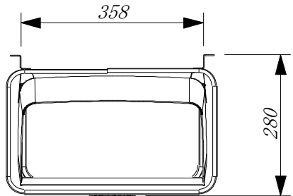
上面図
